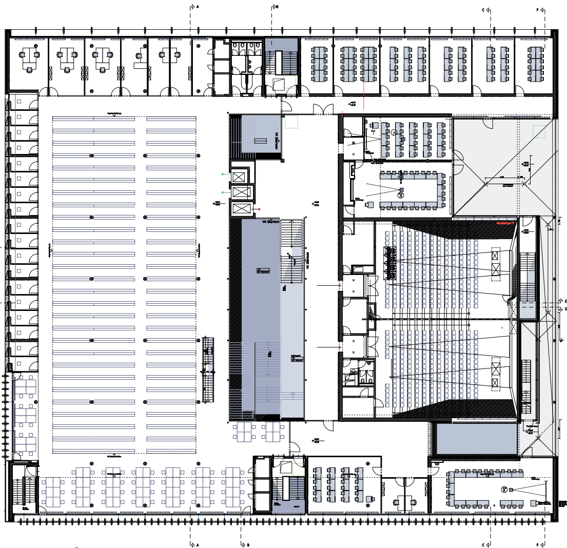
Grundriss 3.OG. ohne Maßstab
